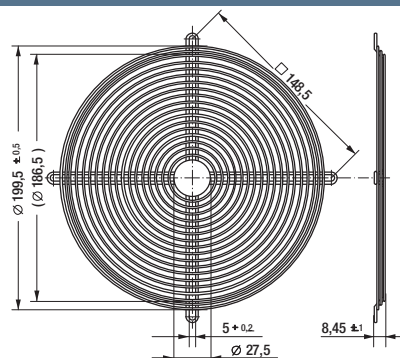
LZ22 Lüfterbaugröße 200 x 51
