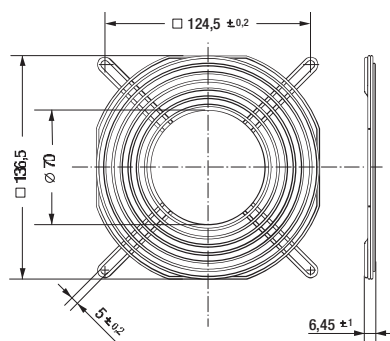
LZ53 Lüfterbaugröße 140 x 140
