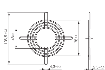
LZ22-2 Lüfterbaugröße 80 x 80
